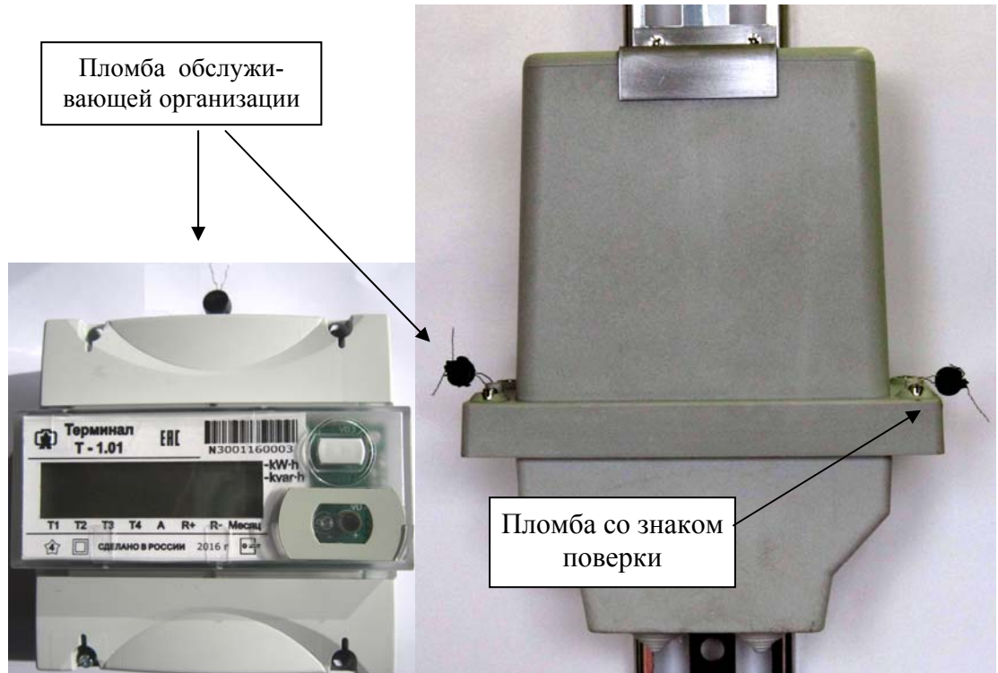
Рисунок 2 – Внешний вид счётчика наружной установки и схема пломбирования
