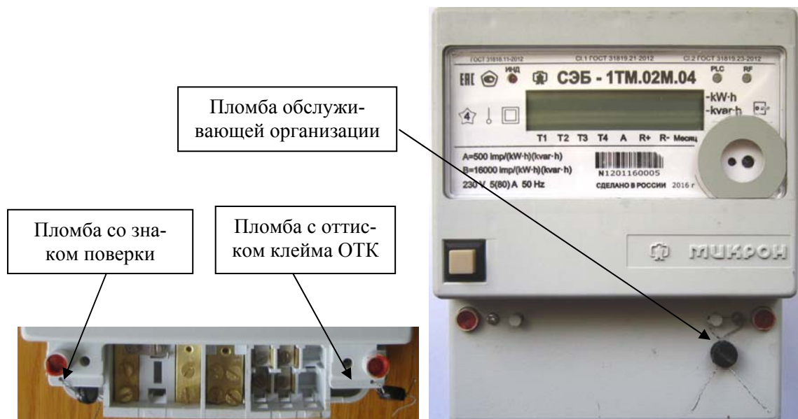
Рисунок 1 – Внешний вид счётчика внутренней установки и схема пломбирования
