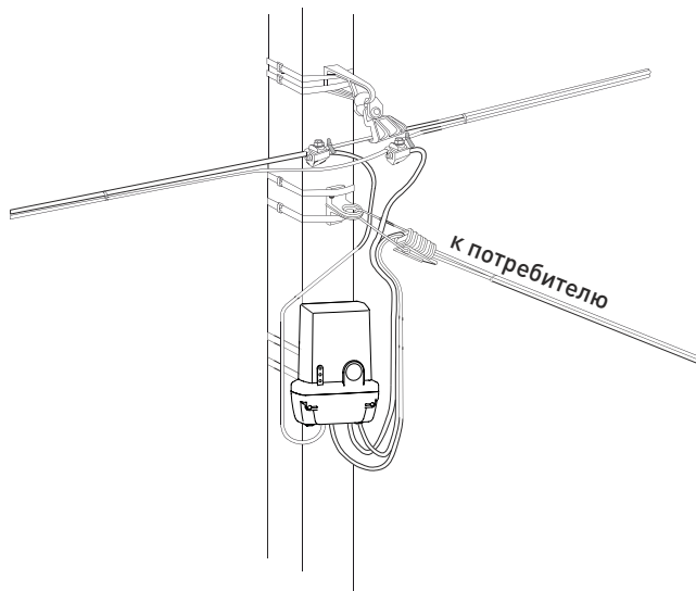
Рисунок 3.1 – Установка измерительного блока на опору линии электропередачи
